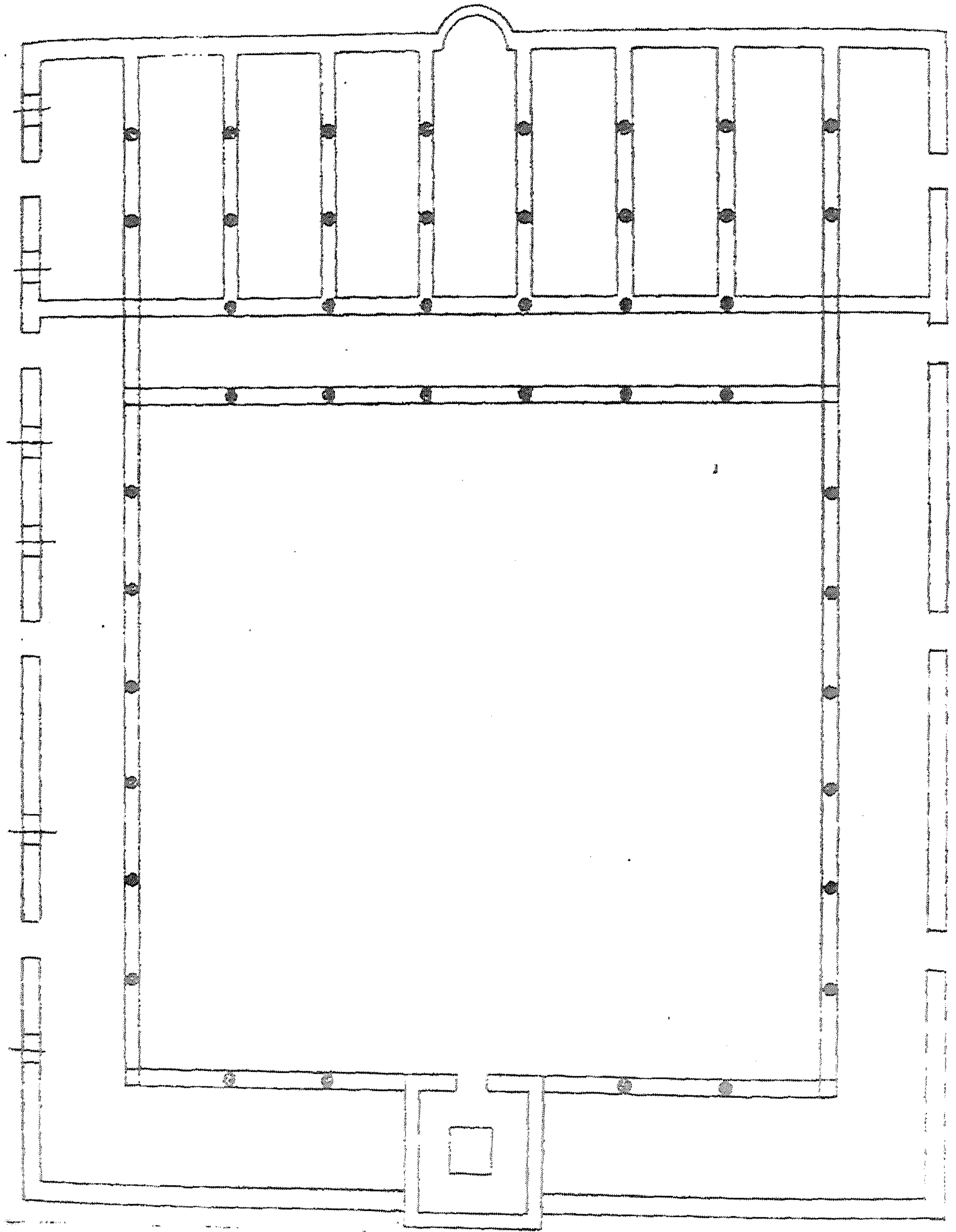
(شكل رقم ٣٩) رسم تخطيطي لجامع صفاقس في عهد الأغالبية كما تصوره كل من مارسية وجولقان
